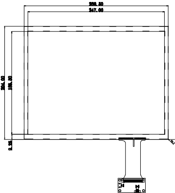
正视图
