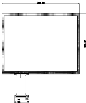
背视图
