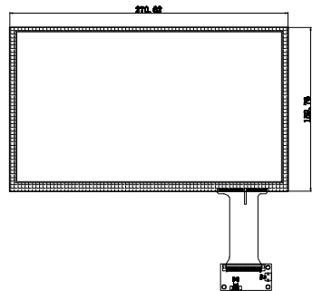
背视图
