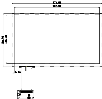
正视图
