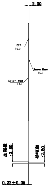
侧视图
