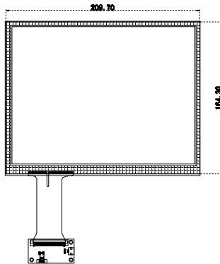
背视图
