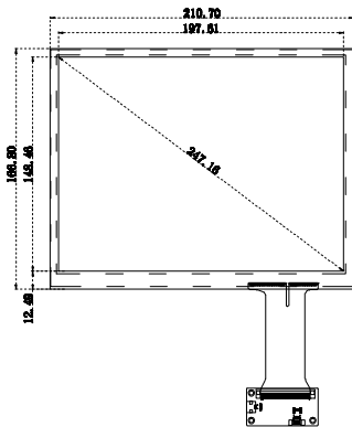
正视图
