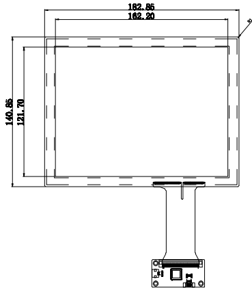
正视图
