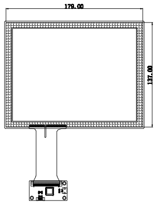
背视图
