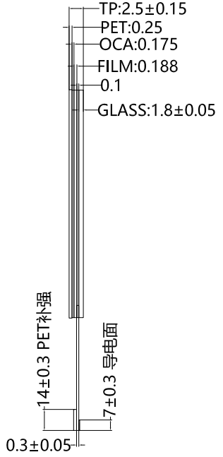
侧视图
