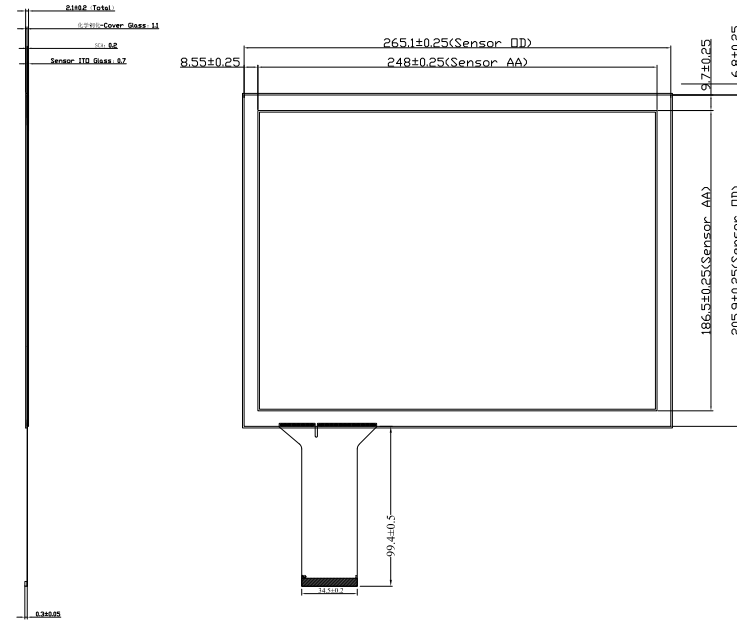
侧视图
