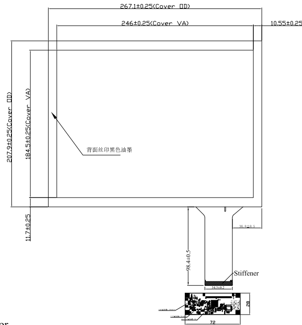
正视图
