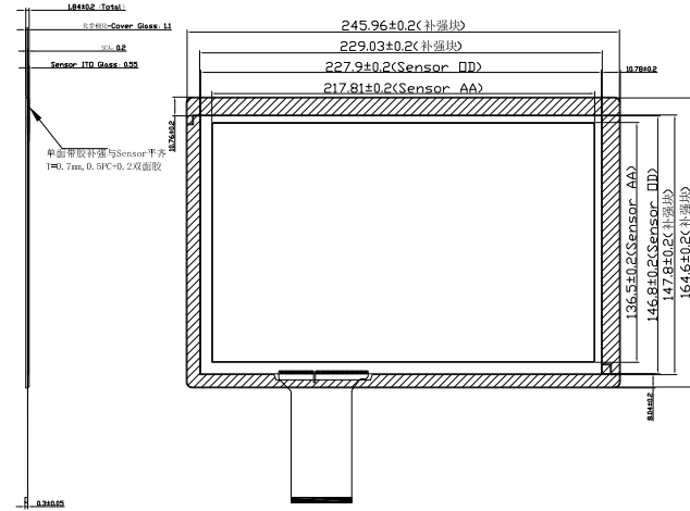
背视图
