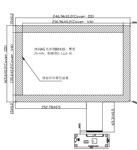
正视图
