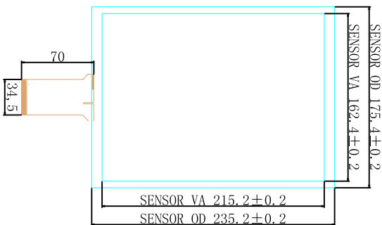
背视图
