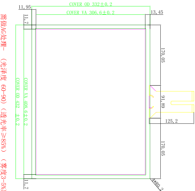
正视图
